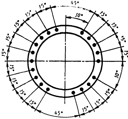
СК26.1—1.5, СК26.1—2.5
