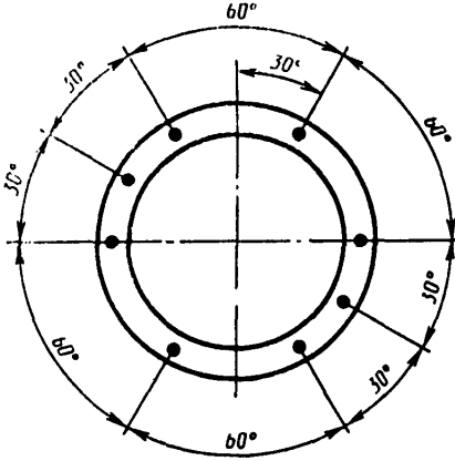
СК26.1—1.5, СК26.1—2.5
