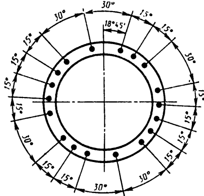
СК22.2—1.2
